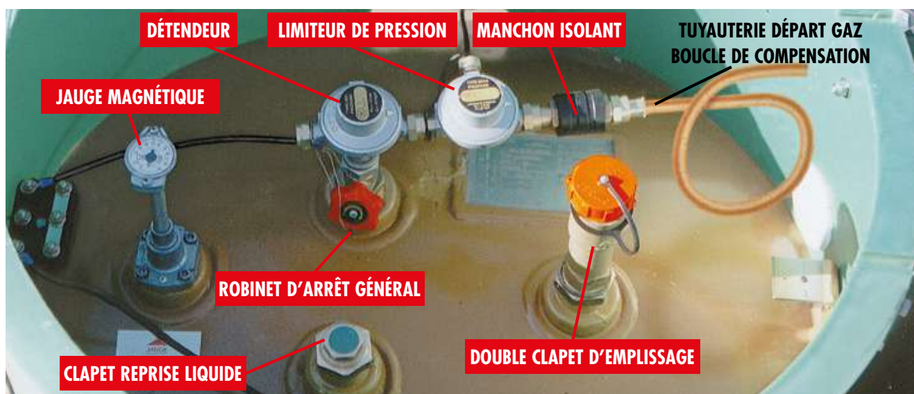
ORGANES SOUS CAPOT DU RÉSERVOIR ENTERRÉ
