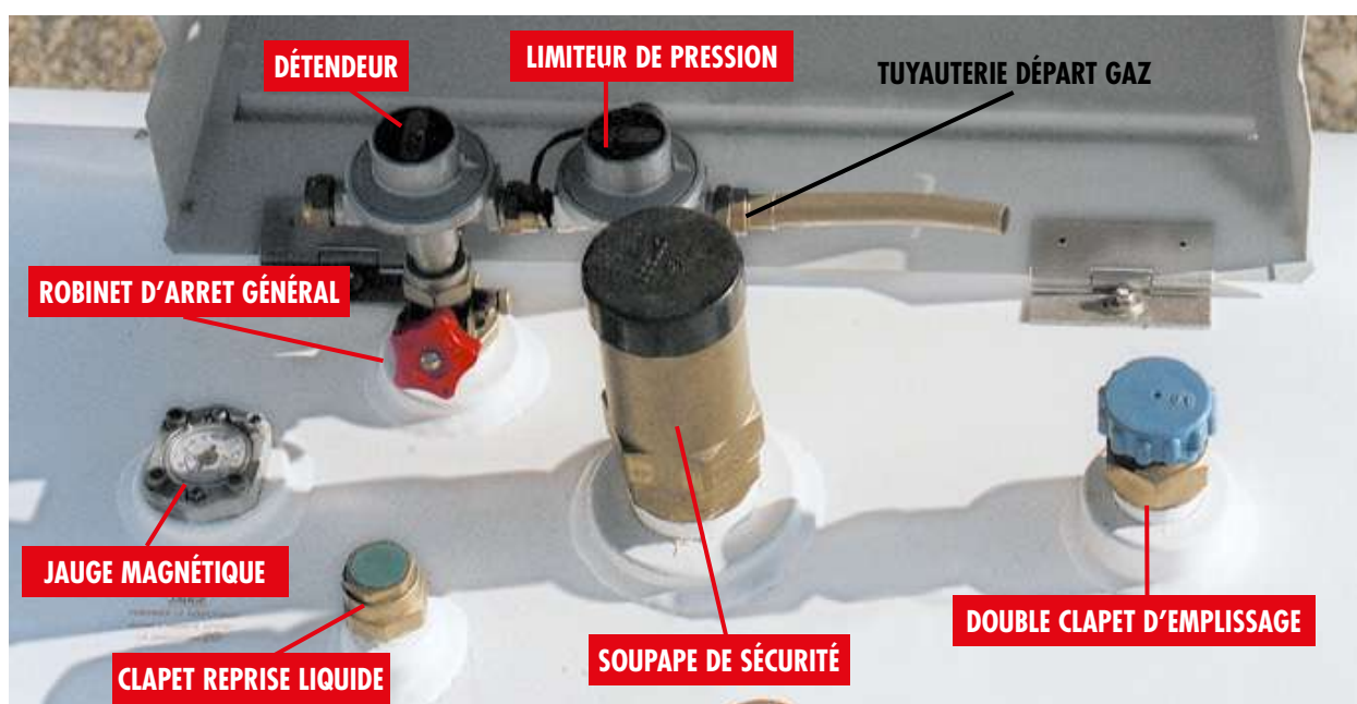
ORGANES SOUS CAPOT DU RÉSERVOIR AÉRIEN
